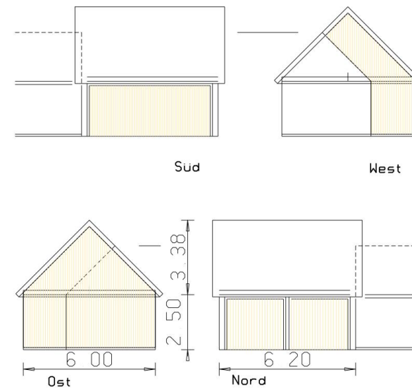
Bauvoranfrage
